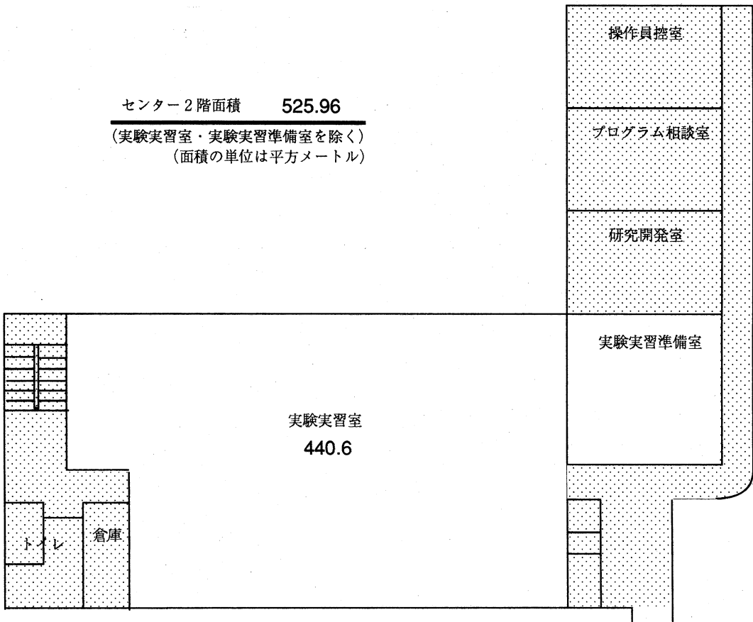
図 1: 飯塚センター 2 階平面図
